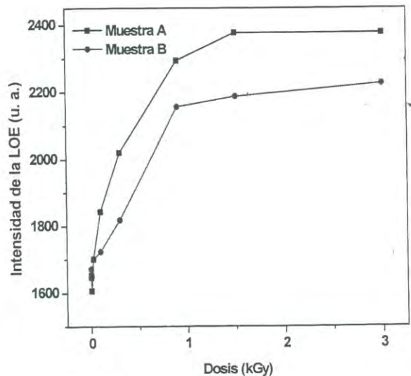
Figura 49. Intensidad LOE contra dosis de irradiación para muestras A y B.
