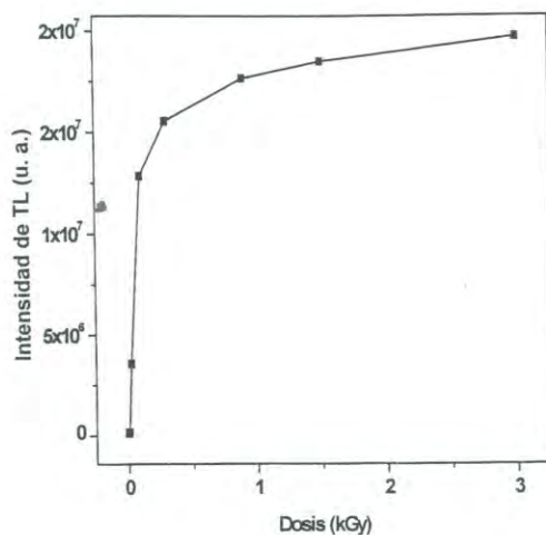
Figura 45. Dosimetría TL sin filtro para la muestra B.
