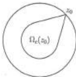
Figura 4.1: Región de convergencia no tangencial
